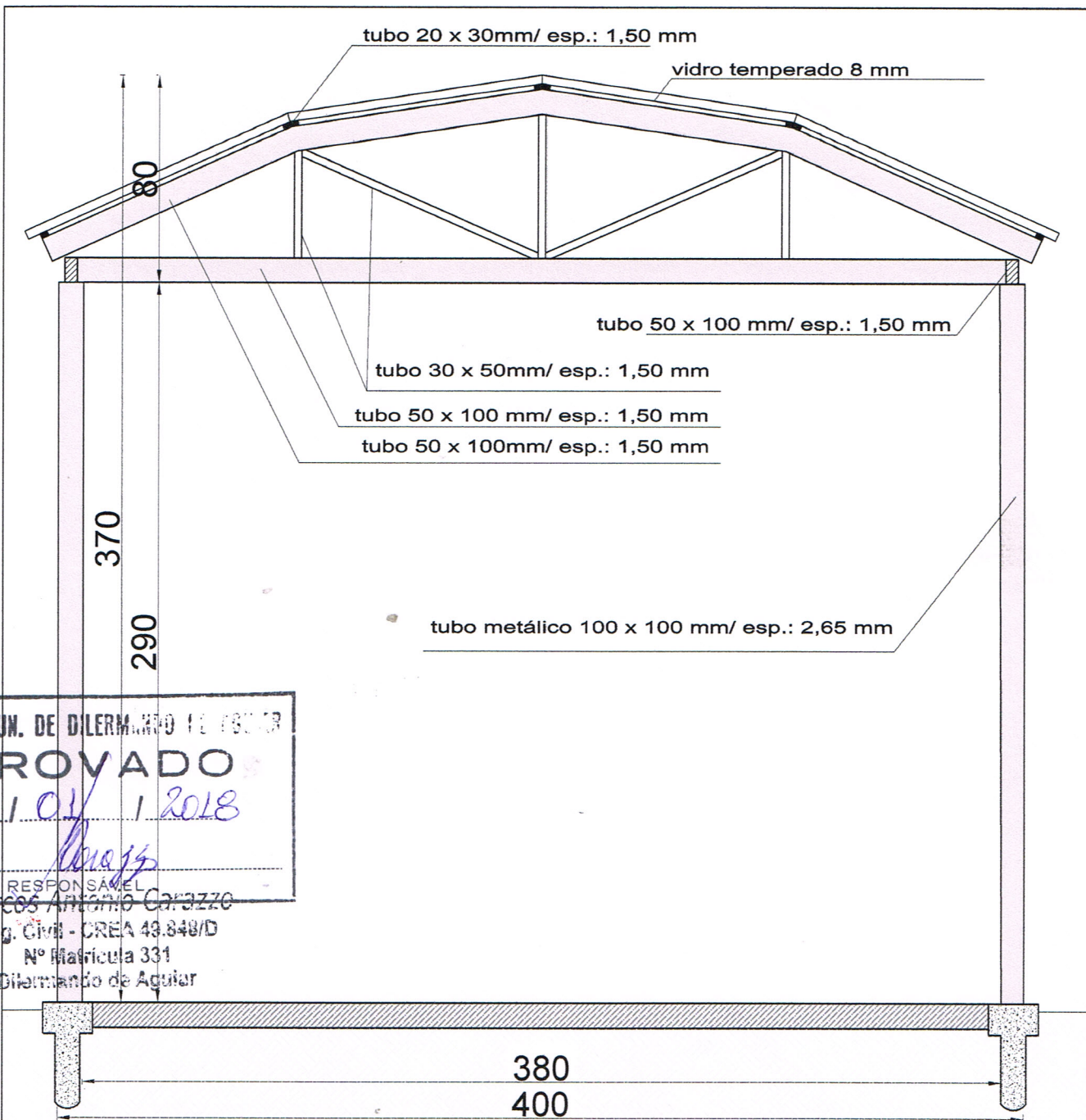
Detalhamento 01 - Cobertura (Escala: 1/25)
